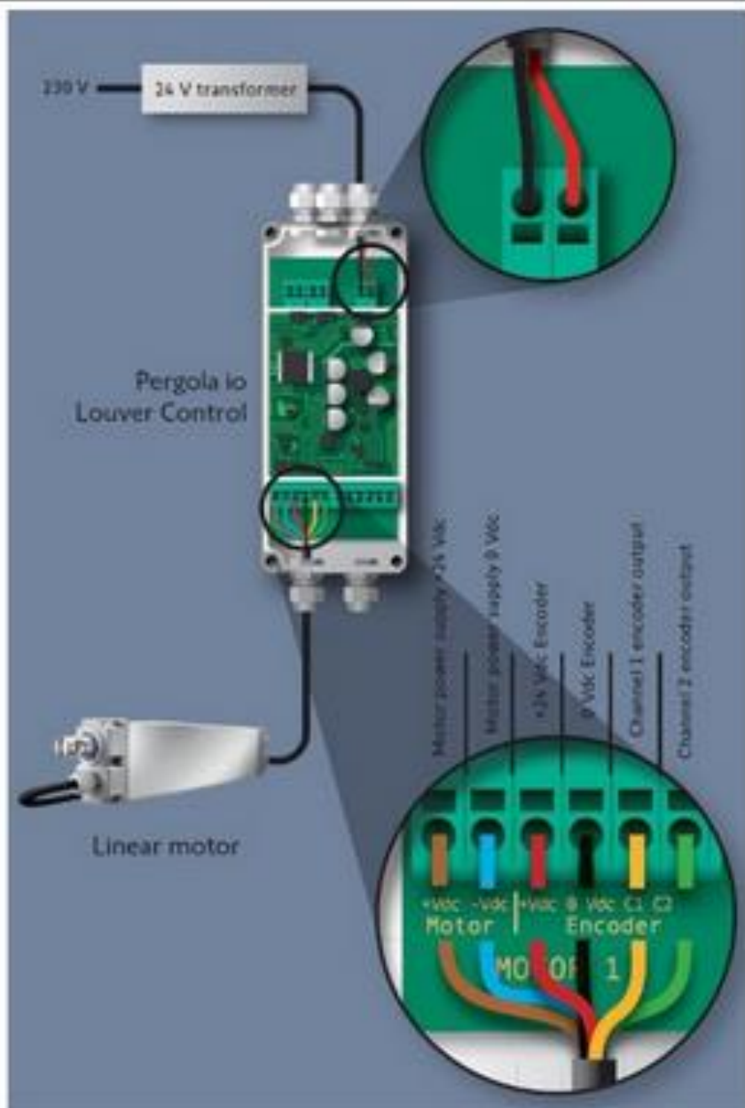
Rys. 35 Schemat obszarów podłączeń wewnątrz centralki Pergola io Louver
