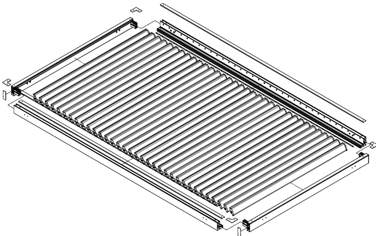
Rys. 6 Widok montażu elementów Pergoli SB400PRO R z dwoma rynnami.
