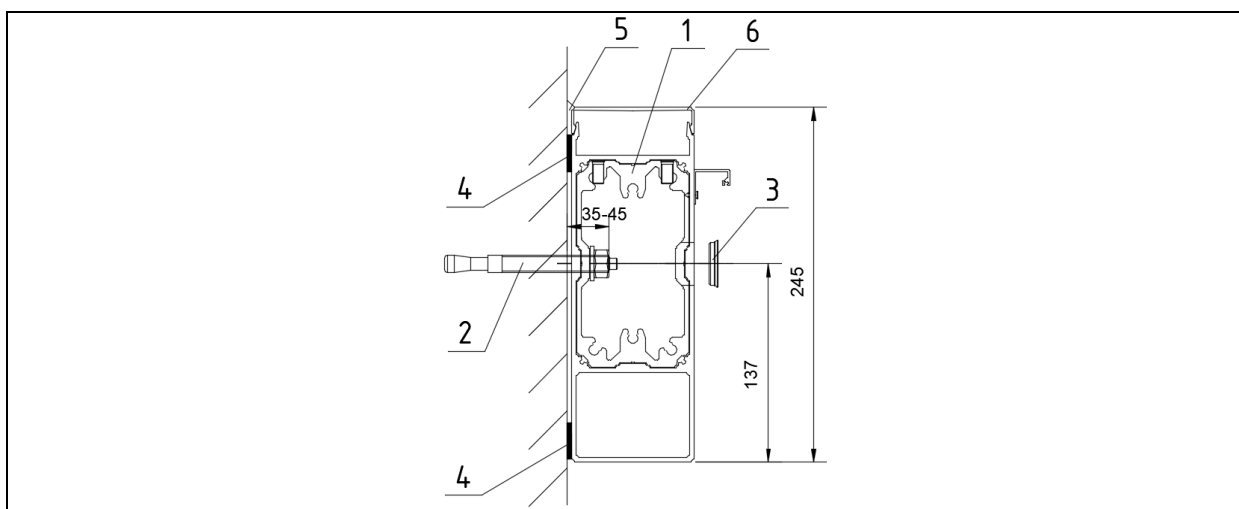
Rysunek 5 – Mocowanie przelotowe (1- łącznik wzmacniający mocowania przyściennego, 2- kotwa M12 (poza dostawą SELT), 3-zaślepka lakierowana, 4-pas taśmy EPDM, 5-uszczelniczącym uszczelniaczem, 6- rewizja belki).
